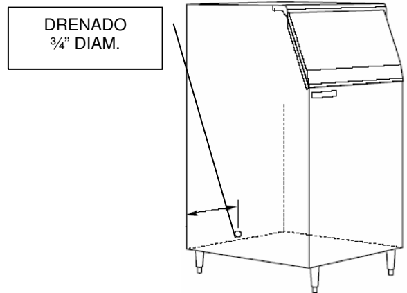
Depósitos DH160, DH250, DH415
